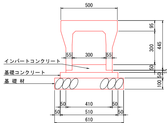
自由勾配側溝 材料表
